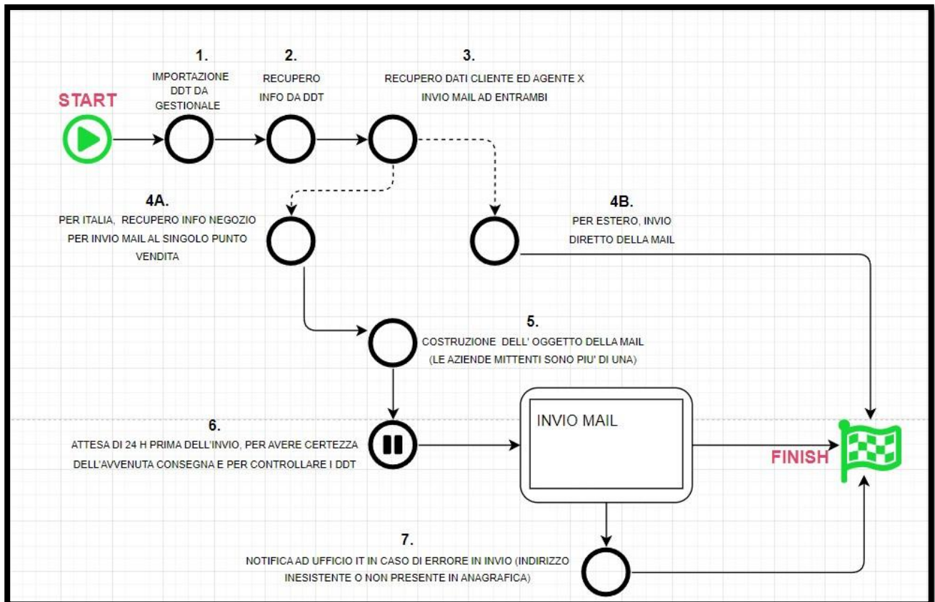
Diagramma del work-flow Arxivar realizzato per Ellepi
